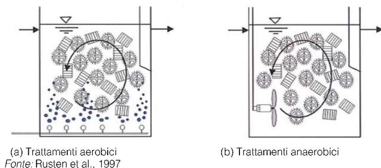
Figura 3.13 – Schema di un processo MBBR.
